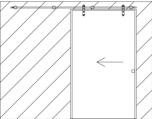
3 ΜΟΝΟΦΥΛΛΗ ΣΥΡΟΜΕΝΗ ΠΟΡΤΑ - ΤΟΙΧΟΣ
