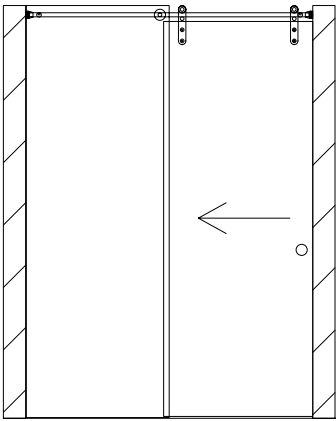
1 ΜΟΝΟΦΥΛΛΗ ΣΥΡΟΜΕΝΗ ΠΟΡΤΑ - ΜΕ ΕΝΑ ΣΤΑΘΕΡΟ ΚΡΥΣΤΑΛΛΟ
